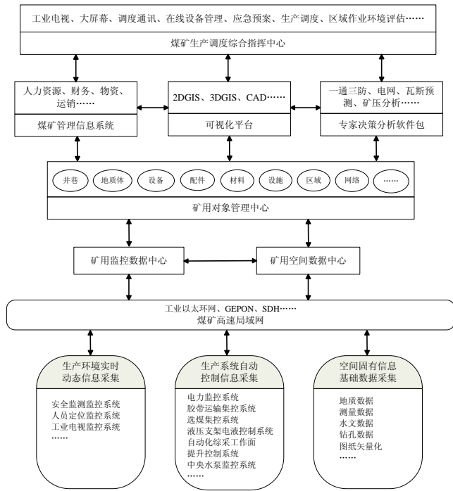
图1 数字矿山建设框架图
